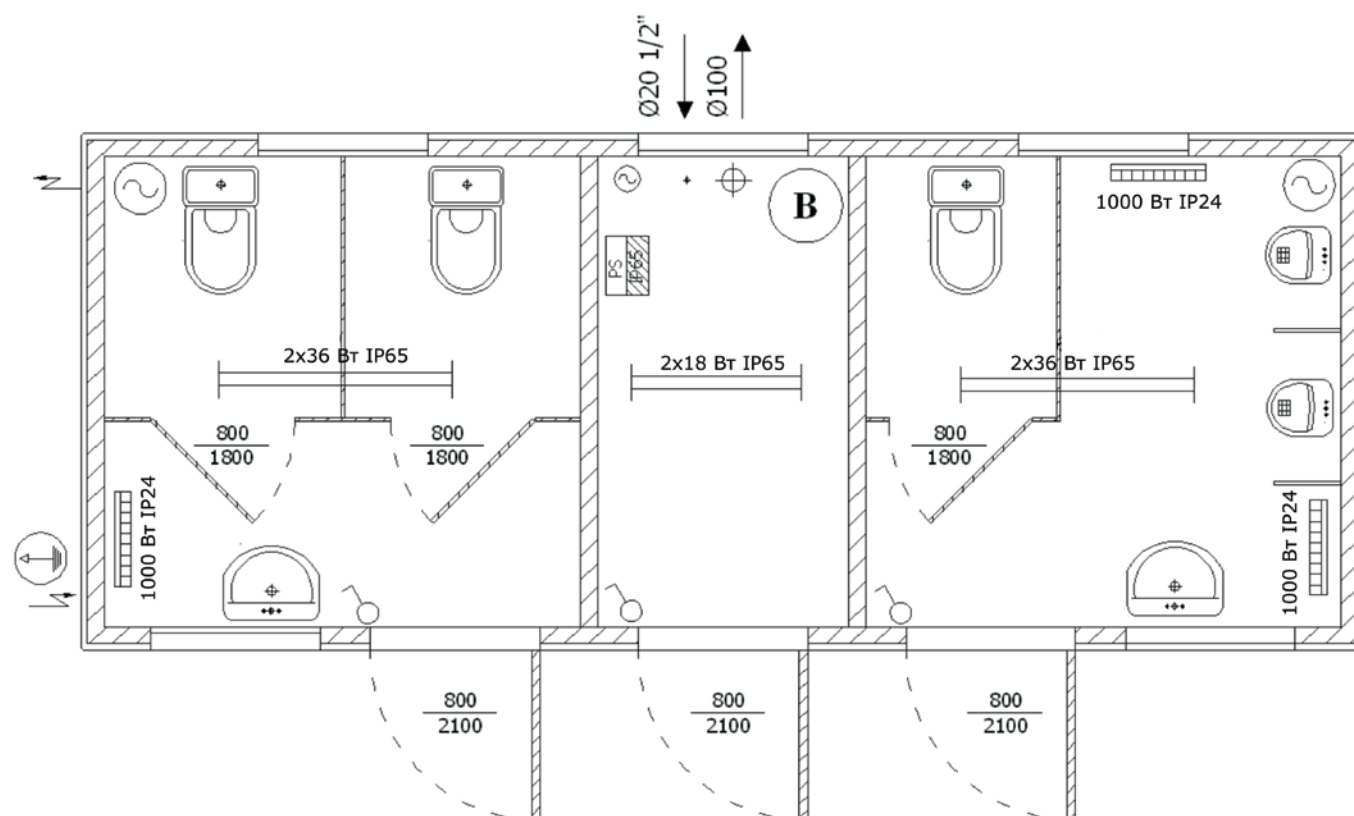
Пример типовой планировки санитарного контейнера
